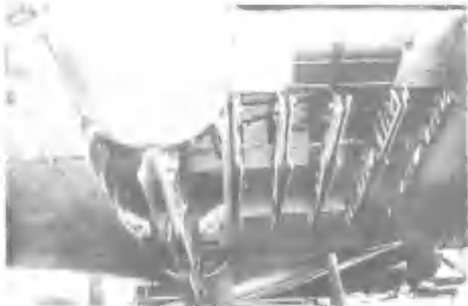
Крыльевые и фюзеляжные бомболюки "Лося", проходившего обследование на заводе N156.
